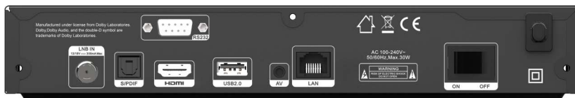
az AB CryptoBox 800HD hátsó panele 2. kép
